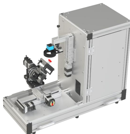
多面画像検査ユニット N-VisionSystem
