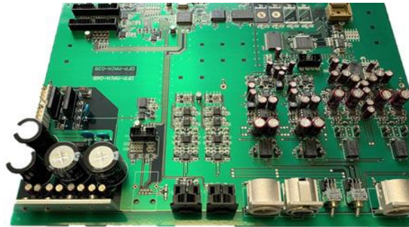
音響機器用基板実装
