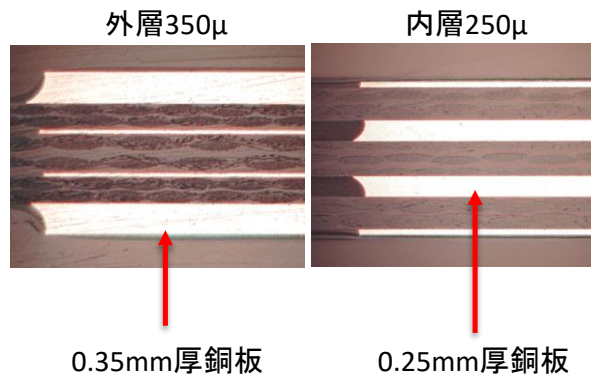
大電流対応基板の断面図
