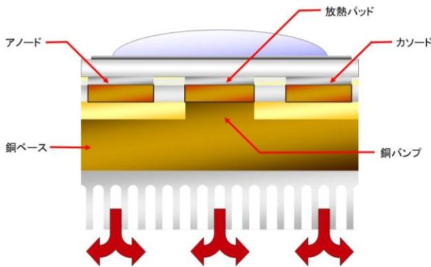
高輝度LED用銅ベース基板の構造
