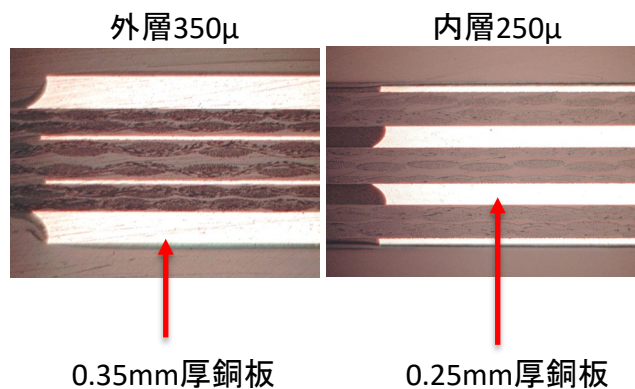
大電流対応基板の断面図
