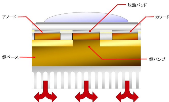
高輝度LED用銅ベース基板の構造
