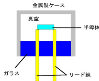
ガラス気密封着イメージ
