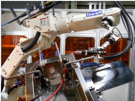
溶接ロボット(Tig溶接)
