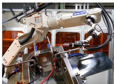
溶接ロボット(Tig溶接)
