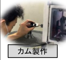
きさげ作業
