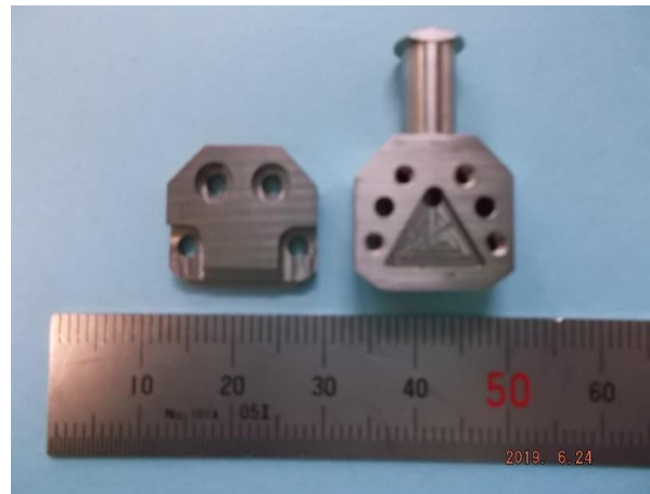
材質: SUS304 微細加工 M2タップ
