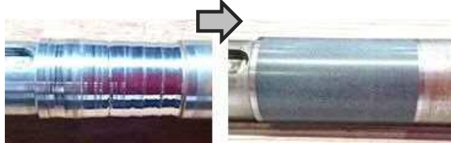
【再生】摩耗したシャフトのシール部:溶射による耐摩耗再生
