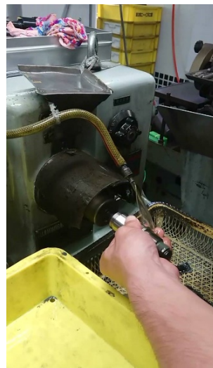
ホーニング加工 (FK-8: 富士ホーニング工業)
