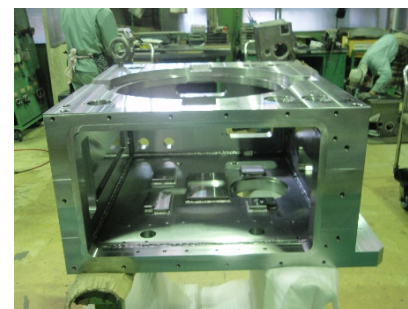
角形真空チャンバ
