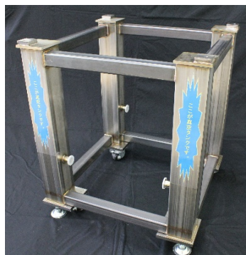
真空タンク付フレーム
