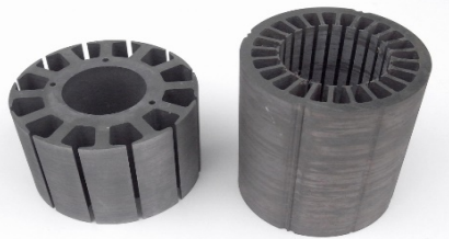
3個取り加工
