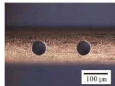
黄銅線, 直径150μm 電極: タングステン, φ50μm 加工時間(各穴): 90秒
