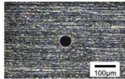
SUS304, 厚さ100μm 電極: タングステン, φ50μm
