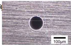
リン青銅, 厚さ 100μm 電極: 黄銅φ100μm
