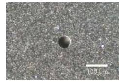
PCD, (穴深さ55μm) 電極: タングステン, φ50μm 加工時間: 3分
