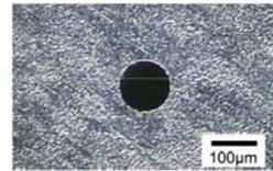
カッター刃, 厚さ 500μm 電極: 黄銅, φ100μm
