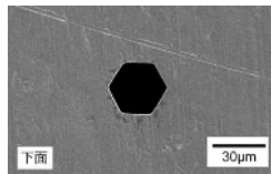
SUS304, 厚さ50μm 電極: 超硬合金 加工時間: 4分
