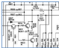
【回路図】
