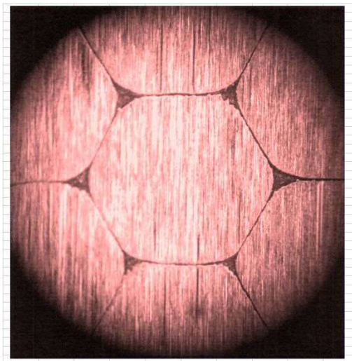
「高密度コイルの断面写真」
