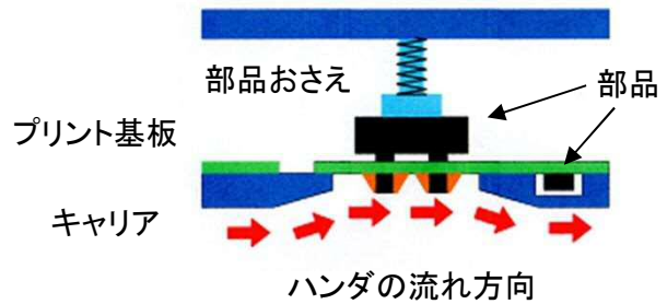
DIPキャリア方式
