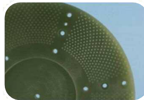
EG(エポキシ)樹脂 φ0.82の微細穴あけ加工
