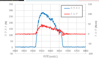
ドリル加工の波形データ
