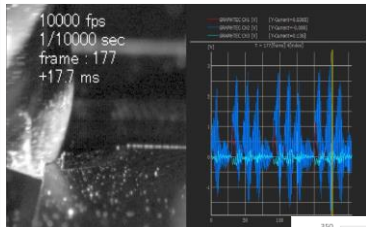
切削動力と高速撮影 (同期再生)
